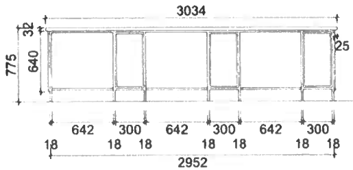
Elevation 01
