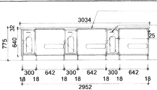
Elevation 02
